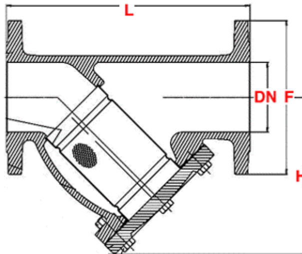
FIG.3011- Dimensioni - Dimensions (mm)
