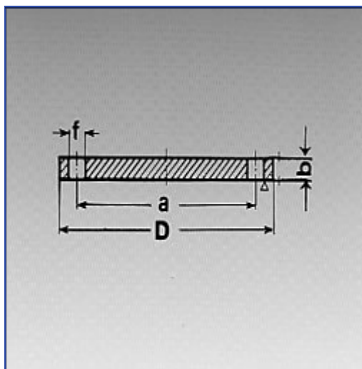
Flange cieche in acciaio PN 25 - PN 40
